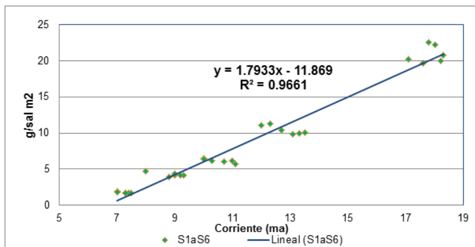
Figura 5. Curva de correlación unificada para todas las soluciones
