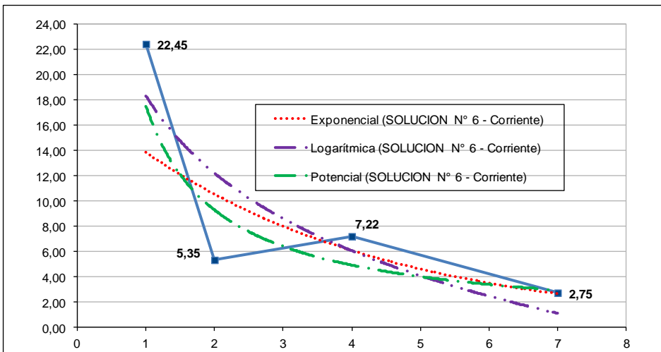
Figura 12. Variación de mediciones de conductividad en el tiempo, soluciones S4 a S6
