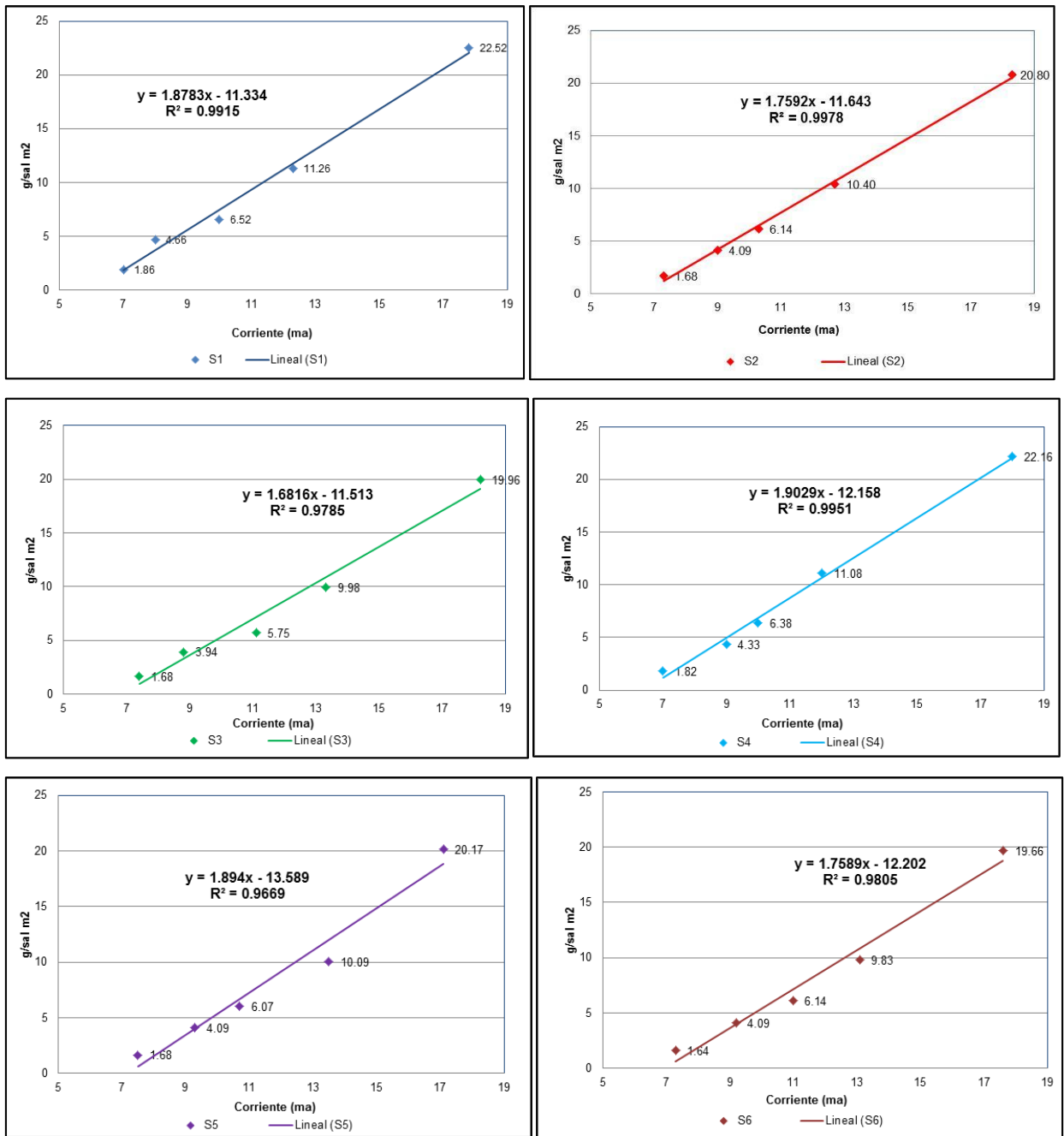
Figura 3. Curvas de calibración de conductividad vs cantidad de sal para las 6 soluciones ensayadas
