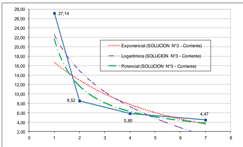
Figura 11. Variación de mediciones de conductividad en el tiempo, soluciones S1 a S3
