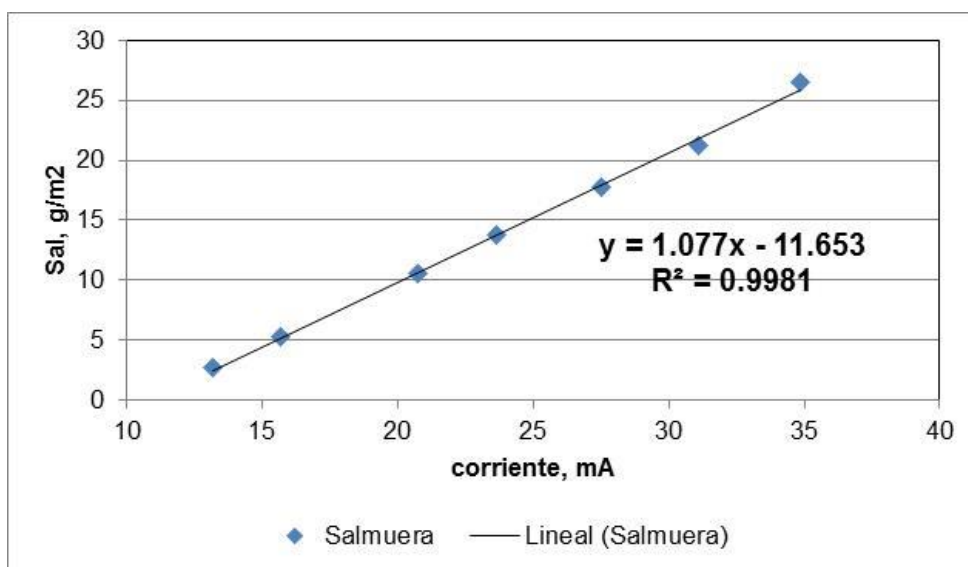
Figura 2. Correlaciones para sal (cloruro de Sodio) disuelta en agua potable
