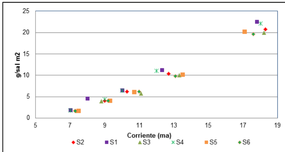
Figura 4. Tendencia de los valores obtenidos para todas las soluciones
